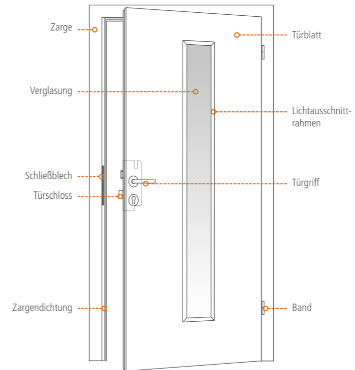
Bestandteile einer Tür/Zarge
